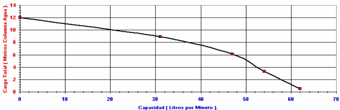
Gasto contra Carga de la Bomba.
