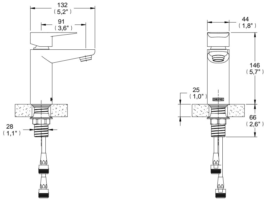
Medidas Referenciales / Estimated Dimensions, Acot.mm.(pulg) / Dim.mm.(in)
