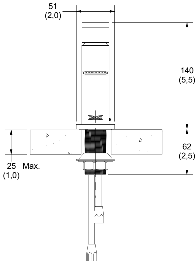
Medidas Referenciales / Estimated Dimensions, Acot. mm [pulg.] / Dim. mm [inches]
