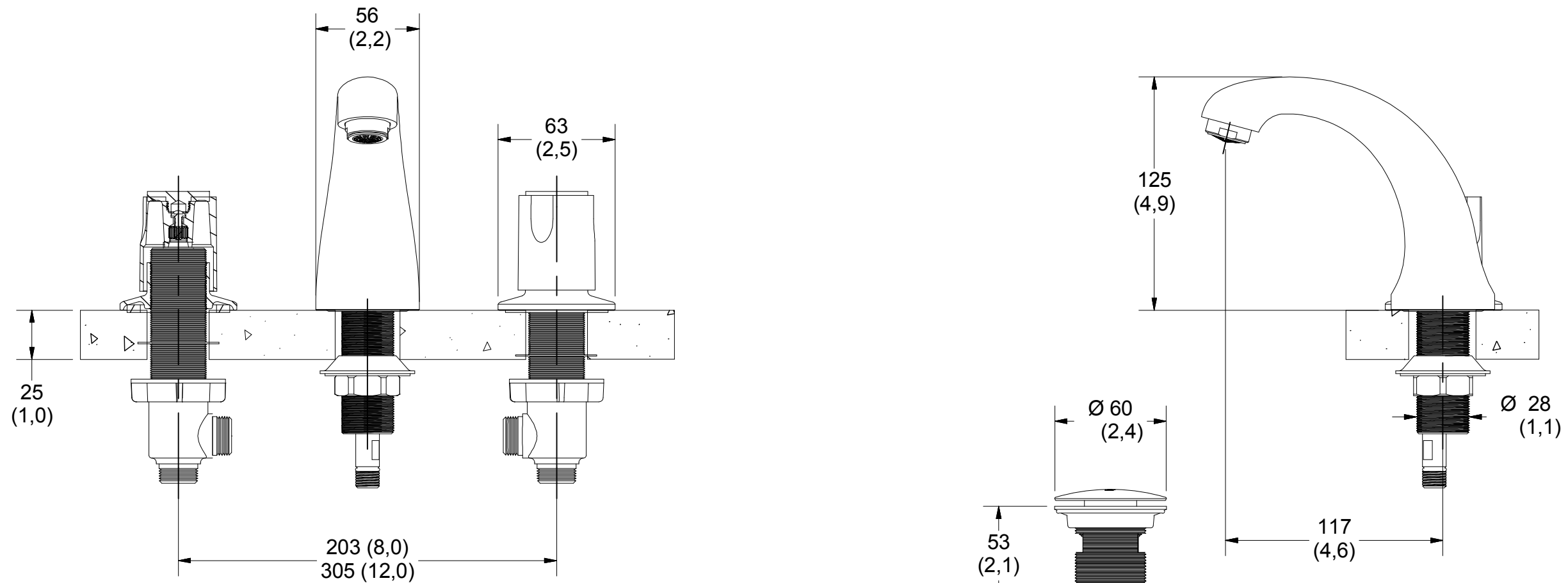
Medidas Referenciales / Estimated Dimensions, Acot. mm [pulg.] / Dim. mm [inch.]
